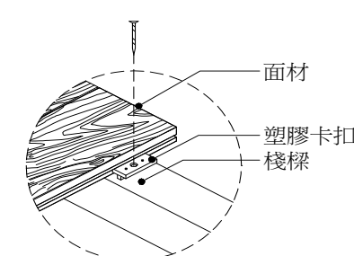
塑膠卡扣固定詳圖
