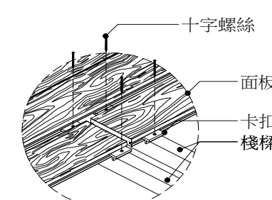
面板交丁處固定詳圖
