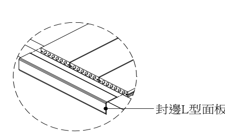
L型收邊條固定詳圖
