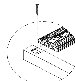
起始板固定詳圖
